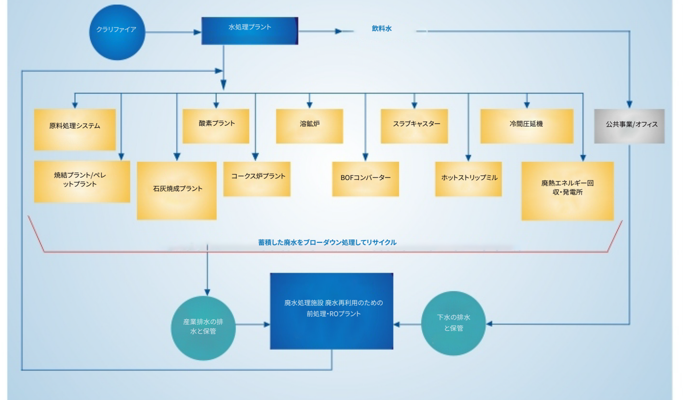
半統合製鉄プラントの一般的な水の流れ図
