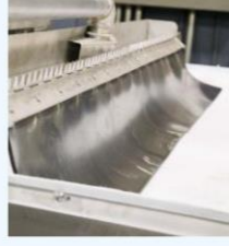
مكبس حزامي لعصرة خام الحديد
