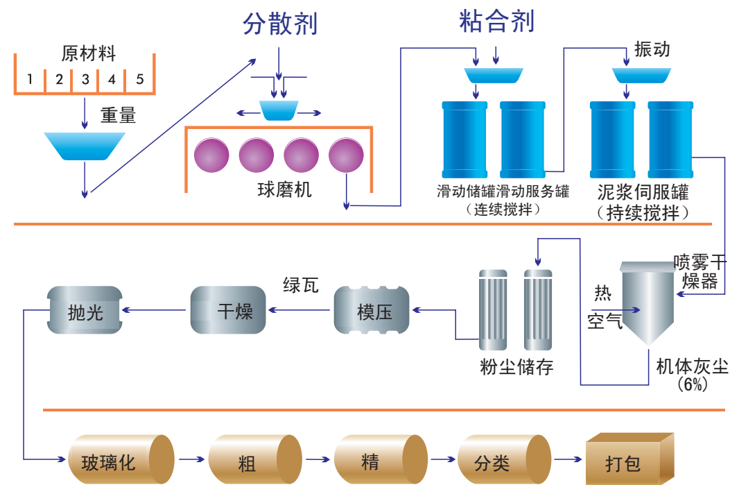
经过验证的制造工艺流程图 INDBOND 粘合剂和 INDION ® 分散剂
